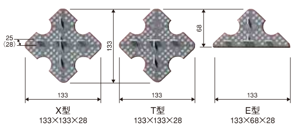
LK20(ロックキーパー20) 歩道及び歩道の車両乗入部
